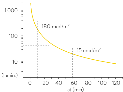
Curva de atenuación del mosaico STARLIGHT* (Resultados obtenidos de nuestros ensayos): Attenuation curve of the STARLIGHT* mosaic (Results obtained in our tests):
